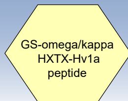
Group 32: ニコチン性 アセチルコリン受容体(nAChR) アロステリックモジュレーター - site II
