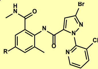
クロラントラニプロール R=Cl シアントラニプロール R=CN
