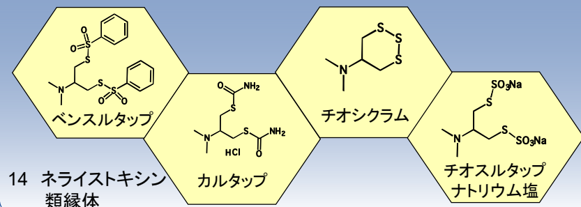
Group 14: ニコチン性アセチルコリン受容体(nAChR) チャンネルブロッカー
