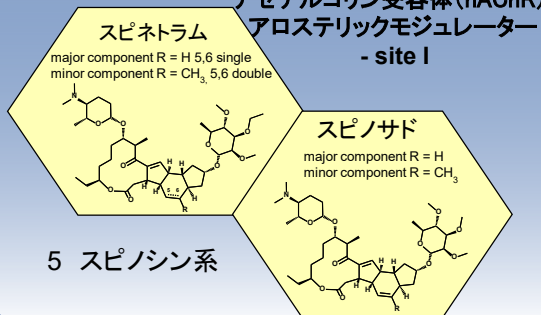
Group 32: ニコチン性 アセチルコリン受容体(nAChR) アロステリックモジュレーター - site II
